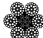
6 x 41 SEALE-FILLER WIRE
