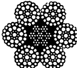
6 x 46 SEALE-FILLER WIRE
