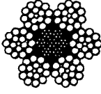
6 x 21 FILLER WIRE
