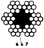
6 x 7
