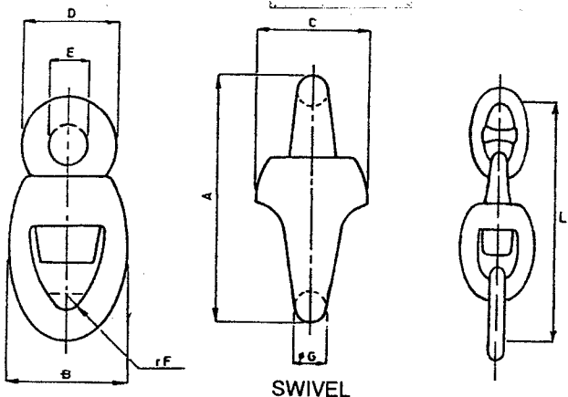
SWIVEL
